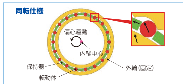
■ 偏心式ローラ減速機挙動メカニズム
